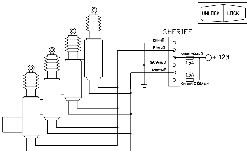
СХЕМА УПРАВЛЕНИЯ ДОПОЛНИТЕЛЬНЫМИ ЭЛЕКТРОПРИВОДАМИ
