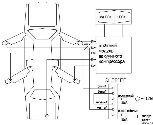
СХЕМА УПРАВЛЕНИЯ ВАКУУМНЫМИ СИСТЕМАМИ «Мерседес-Бенц», «Ауди»
